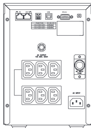
Rückansicht / Rear view 1000 VA / 2000 VA
