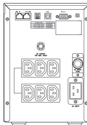
Rückansicht / Rear view 3000 VA
